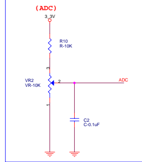
ADC
